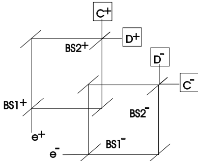
FIG. 1. Hardy’s gedanken-experiment
